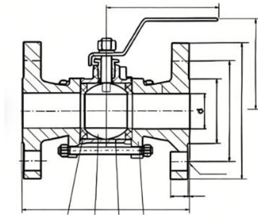
Q41F 法兰三片式球阀结构图
